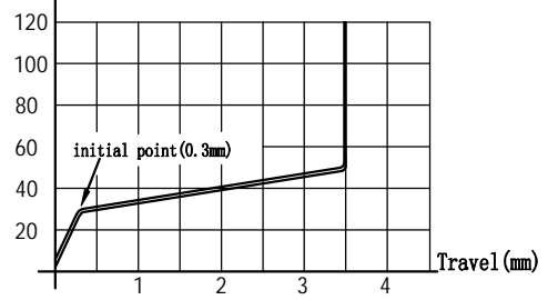
Force-Travel -Diagram
